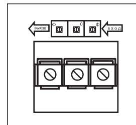
Рис. 6. Клеммник
