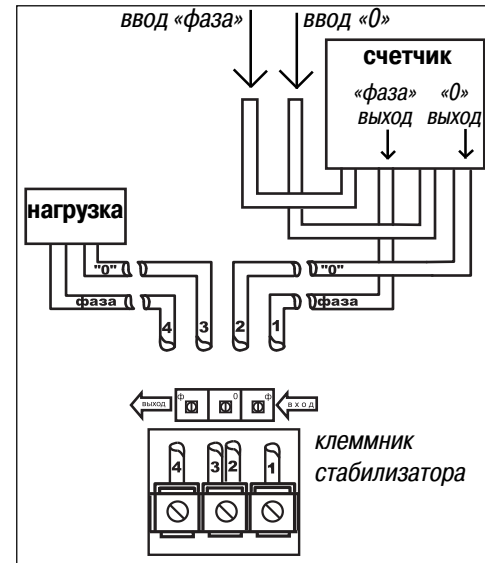
Рис.17. Схема установки
