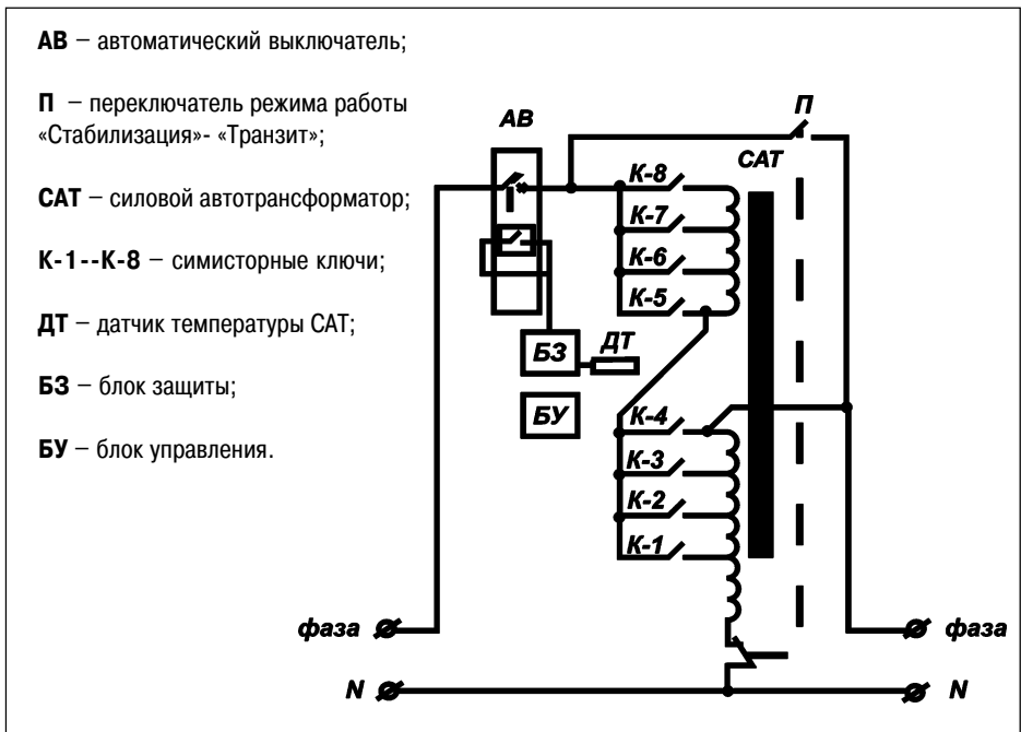
Рис. 9. Структурная схема стабилизатора
