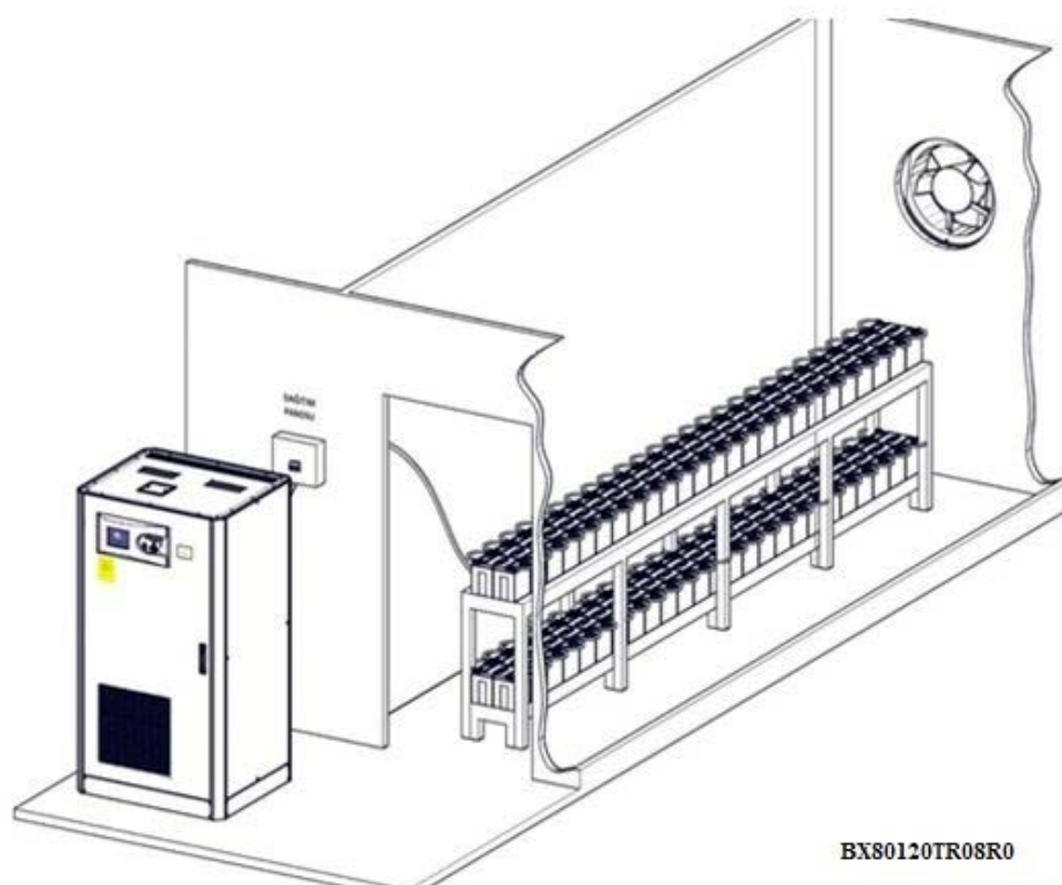
Пример применения помещения для аккумуляторов
