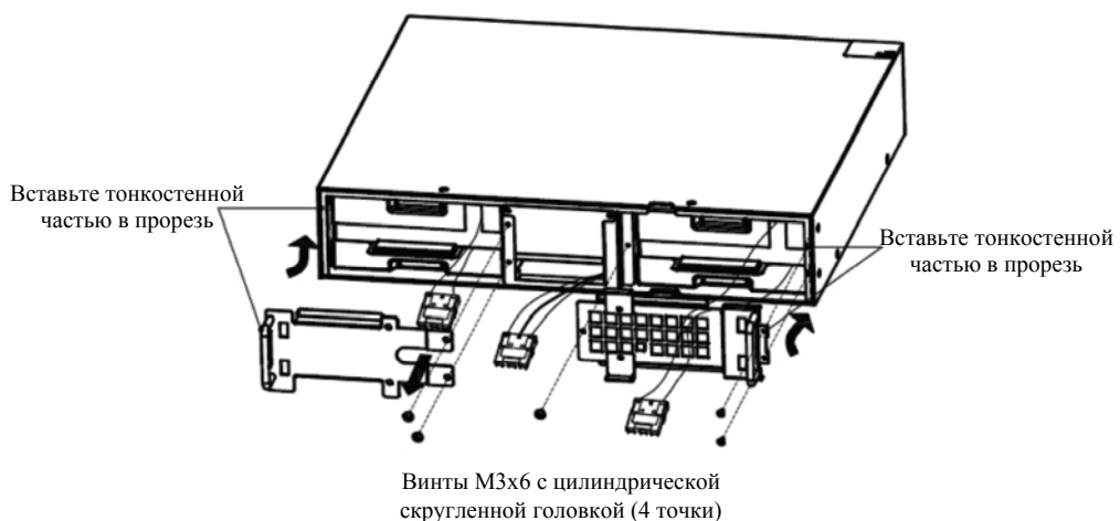
Рис. 28 Установка нового комплекта аккумуляторных батарей
