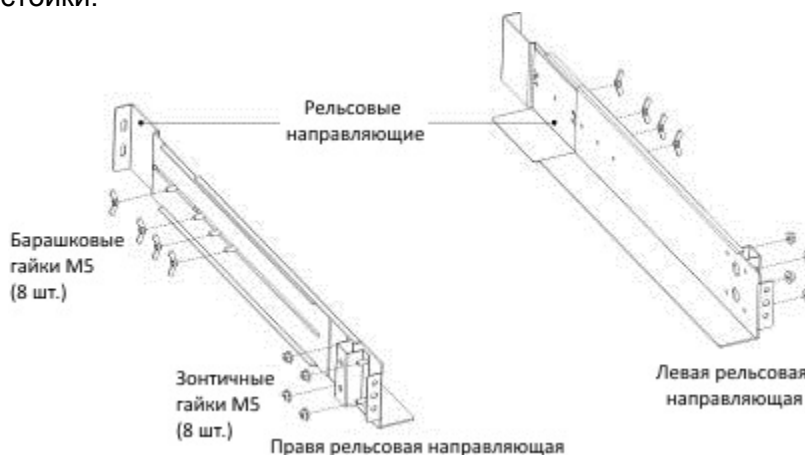
Рис. 4 Крепление рельсовых направляющих
