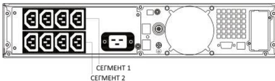
Рисунок 31. 1500/2000 ВА Rack/Tower
