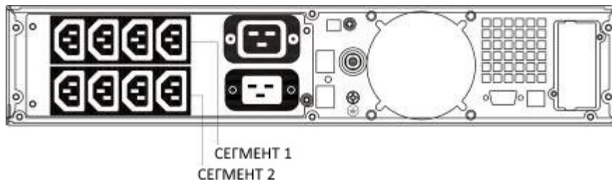
Рисунок 32. 3000 ВА Rack/Tower
