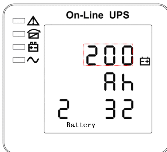
Настройка емкости аккумуляторных батарей (Примечание: Область внутри пунктирной линии будет мигать)
