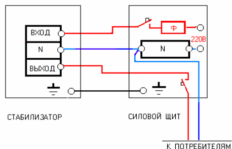
СХЕМА ЭЛЕКТРИЧЕСКИХ СОЕДИНЕНИЙ
