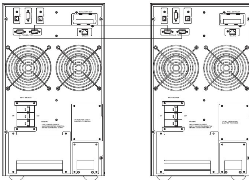
Параллельная система из двух ИБП
