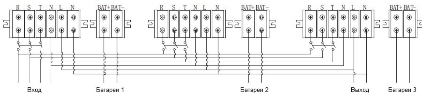
Схема подключения параллельной системы из трех ИБП
