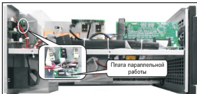
Плата параллельной работы для моделей 6 кВА и 10 кВА
