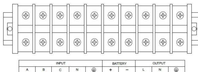
Модели 15 кВа и 20 кВа
