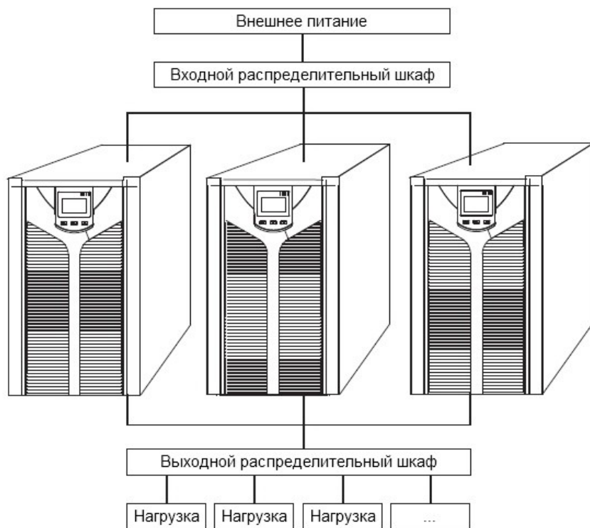
Структурная схема параллельной системы
