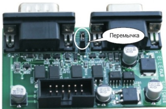
Расположение перемычки
