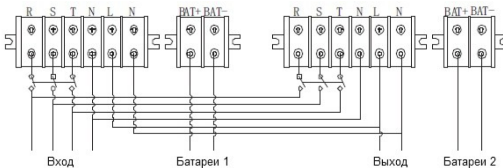
Схема подключения параллельной системы из двух ИБП
