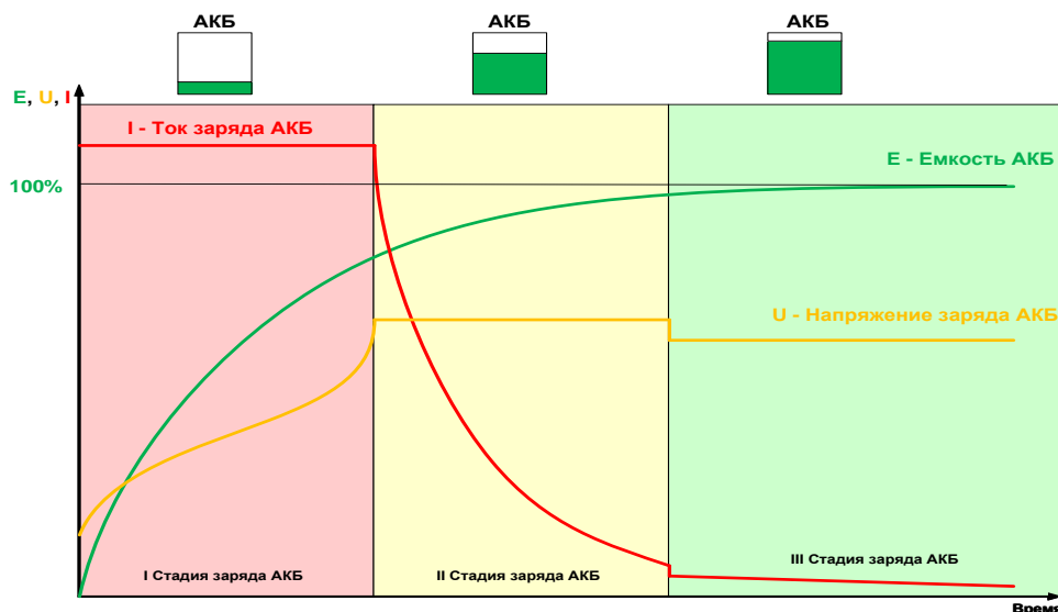
Рис. 4.1 Графическое отображение работы трёхступенчатого зарядного устройства
