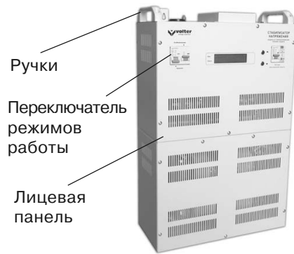
Рис. 1. Стабилизатор напряжения
