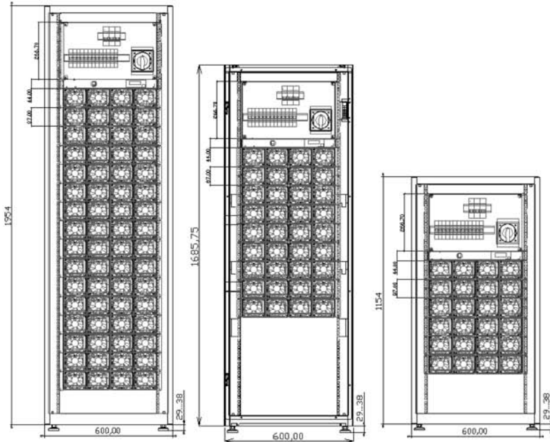
Габаритные размеры основных моделей стабилизаторных систем "Матрикс"
